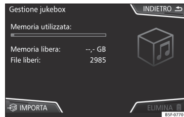
Fig. 25 Gestione jukebox
