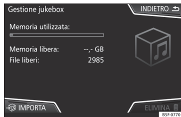
Fig. 42 Gestione jukebox
