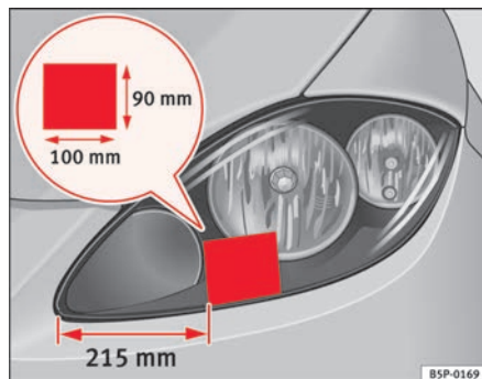
Fig. 151 Faro sinistro
