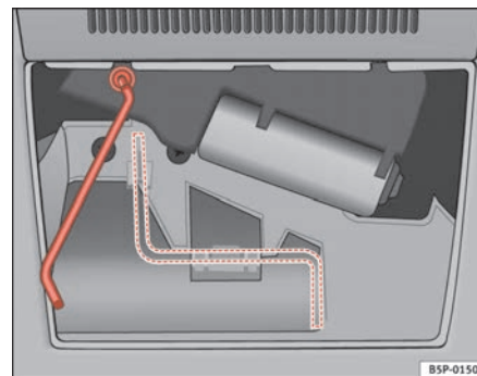
Fig. 72 Manovella chiusura di emergenza
