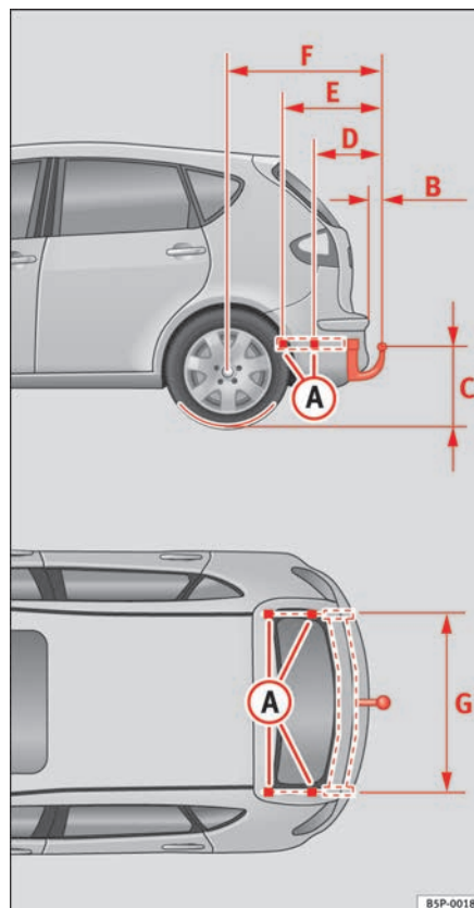
Fig. 158 Punti di ancoraggio per il gancio di traino
