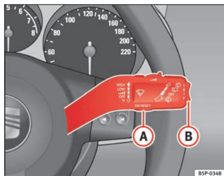
Fig. 45 Leva del tergicristallo: tasto A per la conferma del menu, tasto B per il passaggio ad un altro menu
