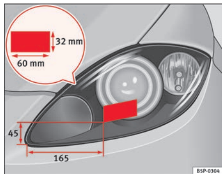
Fig. 157 Faro sinistro
