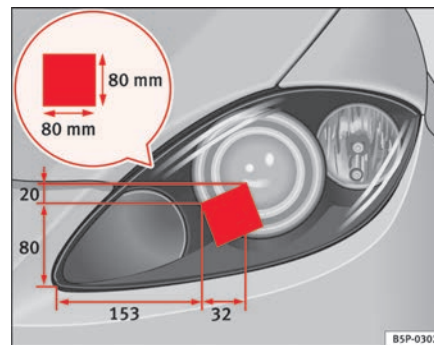
Fig. 155 Faro sinistro
