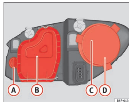
Fig. 182 Lampade del faro principale
