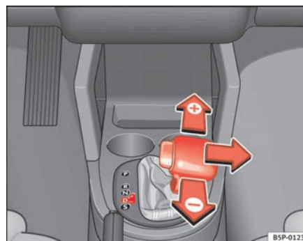
Fig. 142 Cambio del rapporto di marcia con Tiptronic
