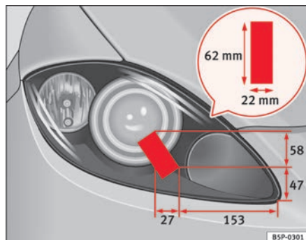
Fig. 154 Faro destro
