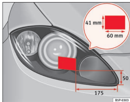
Fig. 156 Faro destro
