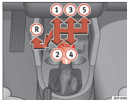
Fig. 136 Dettaglio della console centrale: schema delle marce nel cambio meccanico a 5 rapporti
