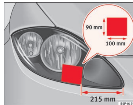
Fig. 152 Faro destro
