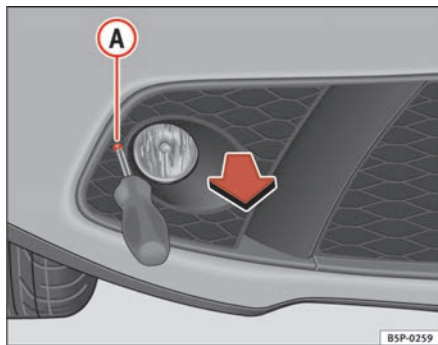
Fig. 205 Accesso alloggiamento occhiello di traino
