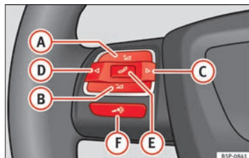
Fig. 45 Comandi sul volante.
