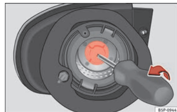
Fig. 187 Indicatore di direzione
