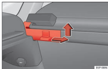
Fig. 106 Smontaggio del pianale portaoggetti.
