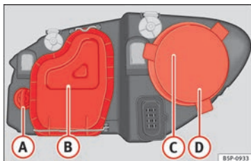
Fig. 176 Lampadine del faro principale.
