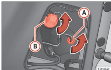
Fig. 192 Luce di posizione.
