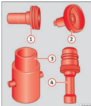
Fig. 142 Quadro generale degli adattatori del bocchettone di riempimento del GPL.
