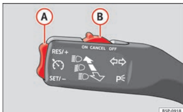
Fig. 135 Leva degli indicatori di direzione e degli abbaglianti: interruttore e tasto doppio del regolatore di velocità.
