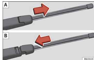
Fig. 171 Sostituzione della spazzola del tergilunotto.
