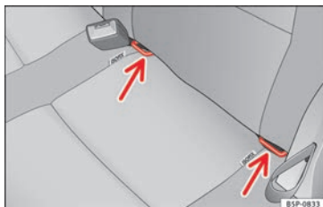
Fig. 23 Occhielli di fissaggio del sistema ISOFIX.
