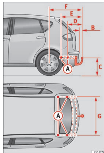
Fig. 138 Punti di ancoraggio per il dispositivo di traino.
