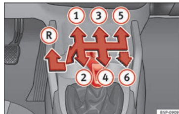
Fig. 124 Dettaglio della console centrale: schema di un cambio manuale a 5 o 6 marce.
