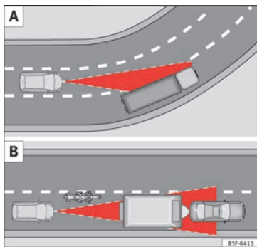
Fig. 184 (A) Veicolo in curva. (B) Motociclista che circola anteriormente fuori dal raggio d'azione del sensore radar.
