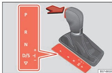
Fig. 168 Blocco della leva selettoria.
