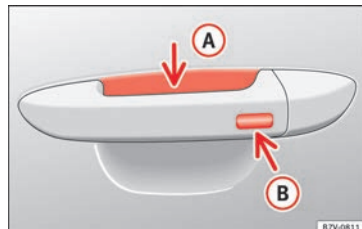
Fig. 126 Sistema di chiusura e avviamento senza chiave Keyless Access: superficie sensibile A di sblocco sulla parte interna della maniglia e superficie sensibile B di blocco sulla parte esterna della maniglia.
