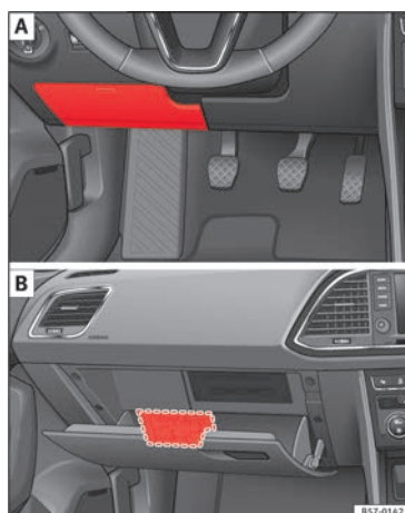
Fig. 64 A Guida a sinistra: coperchio della scatola dei fusibili nella plancia, lato del conducente. B Guida a destra: scatola dei fusibili situata dietro il cassetto portaoggetti.
