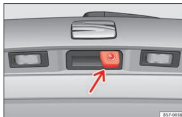
Fig. 233 Nella maniglia del portellone posteriore: posizione della telecamera dell'assistente alla retromarcia.
