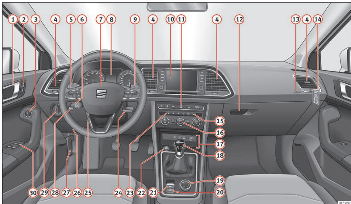
Fig. 118 Postazione di guida.
