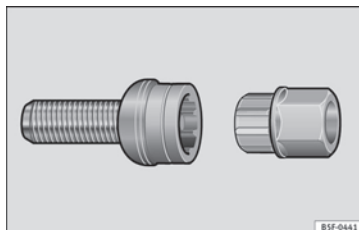
Fig. 73 Vite antifurto con cappuccio ed adattatore.
