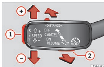
Fig. 189 A sinistra del piantone dello sterzo: terza leva per utilizzare il regolatore di velocità.
