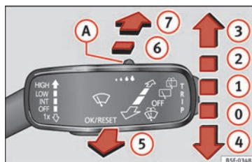
Fig. 40 Uso del tergicristalli e del tergilunotto.
