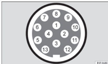
Fig. 236 Rappresentazione schematica: assegnazione dei pin della presa elettrica per il rimorchio.
