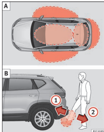
Fig. 131 Sistema di chiusura e avviamento senza chiave Keyless Access: A Zone vicine. B Aprire il portellone posteriore con l'apertura controllata da sensori (Easy Open).
