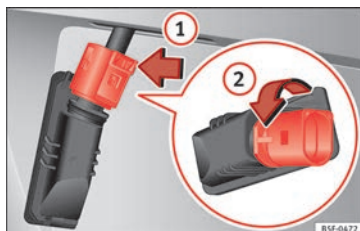
Fig. 116 Luce targa: smontare il portalamпада.
