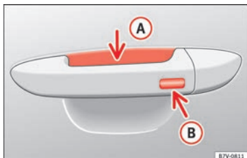
Fig. 132 Sistema di chiusura e avviamento senza chiave Keyless Access: superficie sensibile A di sblocco sulla parte interna della maniglia della porta e superficie sensibile B di blocco sulla parte esterna della maniglia.
