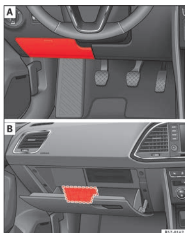
Fig. 66 [A] Guida a sinistra: coperchio della scatola dei fusibili nella plancia del lato conducente. [B] Guida a destra: scatola dei fusibili situata sotto il cassetto portaoggetti.
