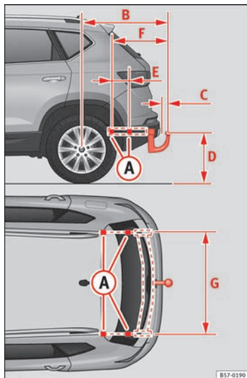
Fig. 237 Quote e punti di fissaggio per il montaggio successivo di un dispositivo di traino.
