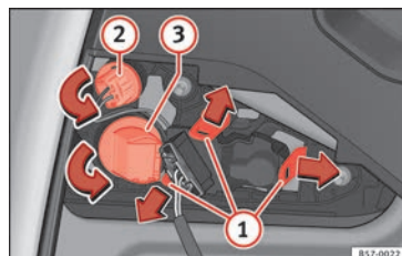
Fig. 114 Smontare il portalamпада.
