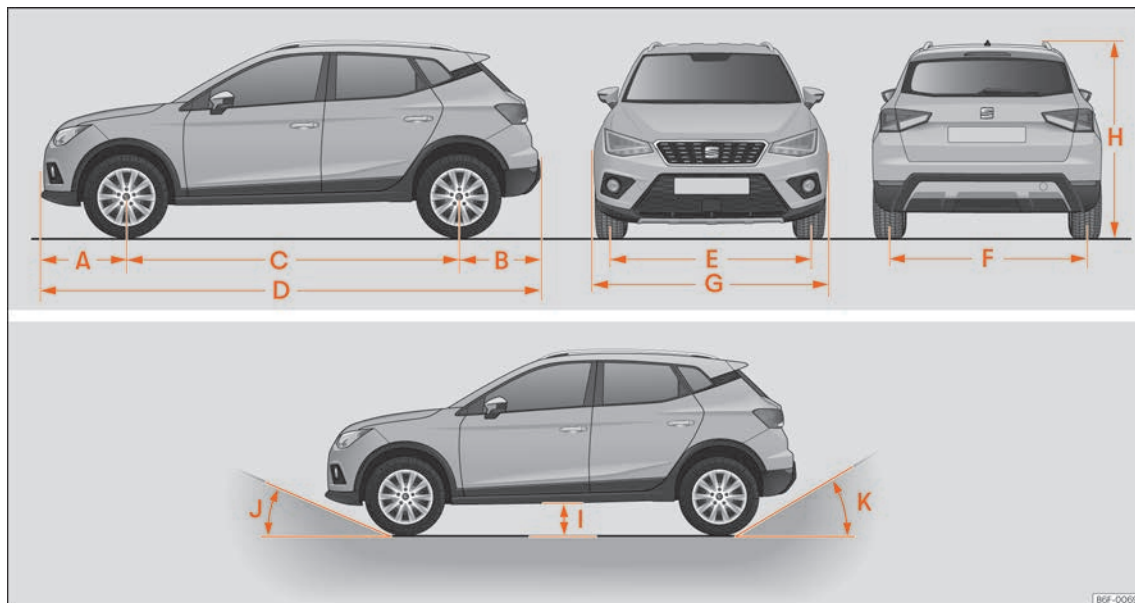
Fig. 289 Dimensioni e angoli.
