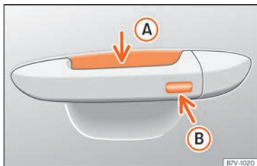
Fig. 139 Sistema di chiusura e avviamento senza chiave Keyless Access: superficie sensibile A di sblocco sulla parte interna della maniglia della porta e superficie sensibile B di blocco sulla parte esterna della maniglia.
