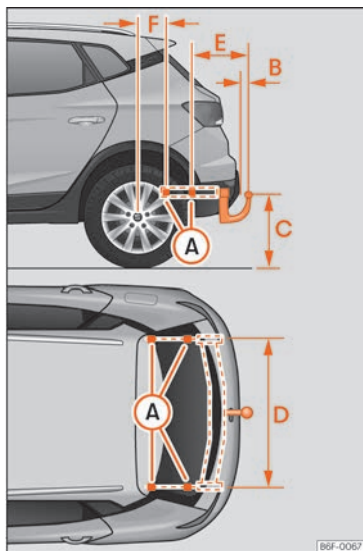
Fig. 276 Punti di ancoraggio per il dispositivo di traino.
