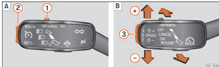
Fig. 50 A sinistra del piantone dello sterzo: A comando e tasti per l'uso del regolatore di velocità; B terza leva per l'uso del regolatore di velocità.
