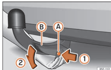
Fig. 273 Estrarre la sfera smontabile
