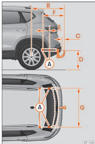
Fig. 300 Quote e punti di fissaggio per il montaggio successivo di un dispositivo di traino.
