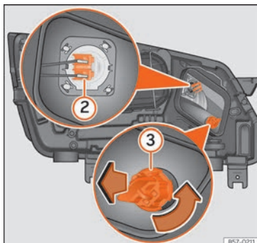
Fig. 111 Nel vano motore: lampadina degli abbaglianti (2) e lampadina degli indicatori di direzione (3).
