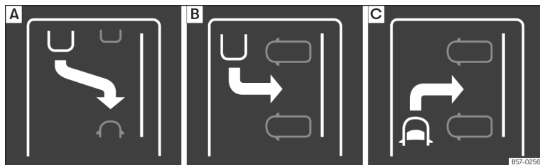
Fig. 281 Quadro generale delle visualizzazioni ridotte per le modalità di parcheggio: [A] Parcheggio in linea in retromarcia. [B] Parcheggiare a pettine in retromarcia. [C] Parcheggiare a pettine con la marcia in avanti.
