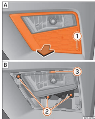
Fig. 112 Faro fendinebbia: estrarre la griglia.
