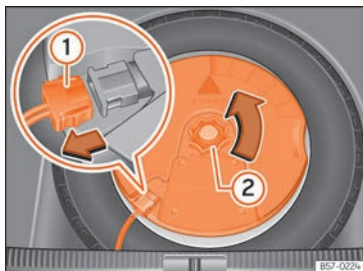
Fig. 312 Nel bagagliaio: smontare il subwoofer.
